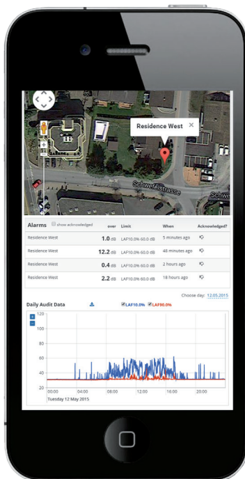
配合 XL2 声级计和 NetBox 在 NoiseScout 网页客户端 实现在线噪声监测
